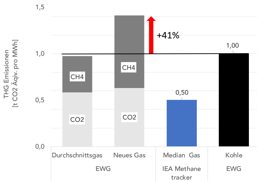
Abbildung 3: Treibhausgasemissionen fossiler Quellen und zusätzliche Emissionen durch die Umstellung von Kohle auf neues Erdgas zur Stromerzeugung: Zusätzliche Methanemissionen überkompensieren etwaige CO 2 -Einsparungen. Quelle: Eigene Berechnungen, IEA Methane tracker.
