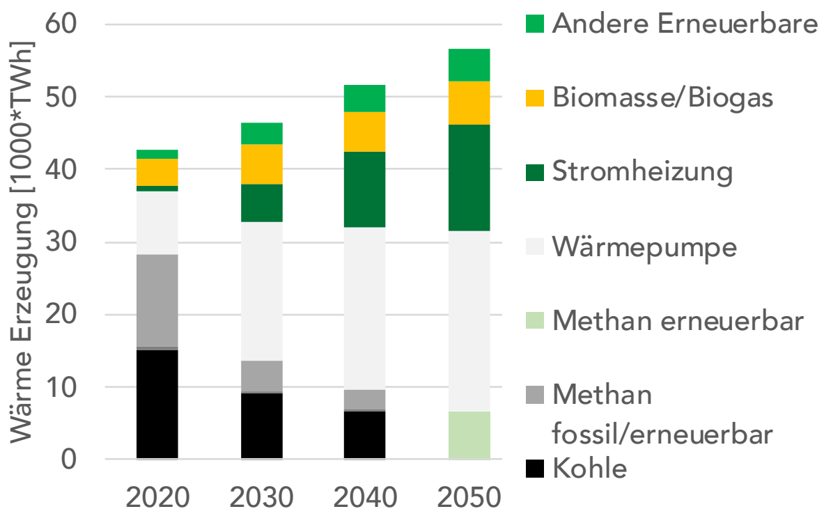
Abbildung 6: Entwicklung der globalen Wärmeerzeugung nach der EWG/LUT-Studie (Ram et al., 2019): Ablösung von fossilem Methan und Kohle vor allem durch Wärmepumpen und Stromheizung. Die Wärmeerzeugung durch Erdölheizungen, die sich im Jahr 2015 noch auf 111 TWh belief, fällt mengenmäßig in der Grafik nicht auf, ist aber insbesondere in Europa durchaus klimarelevant.
