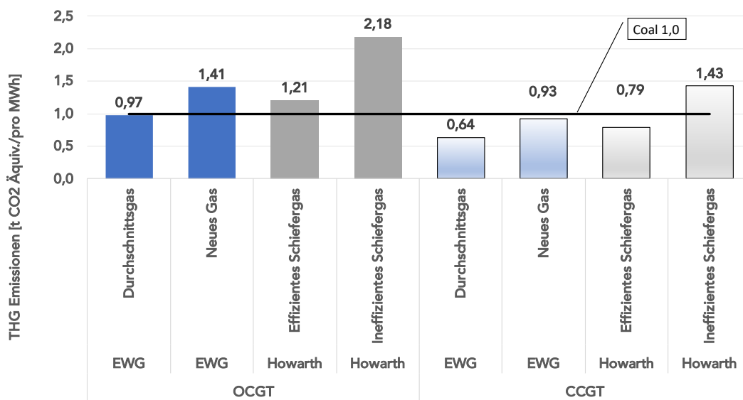
Abbildung 7: Treibhausgasemissionen aus der Stromerzeugung mit Erdgas auf Basis von Lieferkettenschätzungen der EWG für durchschnittliches und neues Gas. Die grauen Balken zeigen die resultierenden Emissionen an, die auf den Emissionen von Schiefergas in der Lieferkette basieren, wie in Howarth (2011) berichtet, jedoch unter Verwendung unserer Annahmen für die Stromerzeugung. Die hellen Farben auf der rechten Seite zeigen die Emissionen teurer GuD-Kraftwerke (CCGT) mit extrem hohem Wirkungsgrad (58%), die in Europa und den meisten Märkten weltweit nicht wettbewerbsfähig sind.
