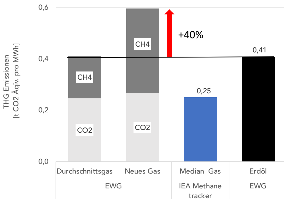
Abbildung 4: Treibhausgasemissionen fossiler Quellen und zusätzliche Emissionen durch die Umstellung von Erdöl auf neues Erdgas zur Wärmeerzeugung: Zusätzliche Methanemissionen überkompensieren etwaige CO 2 -Einsparungen. Quelle: Eigene Berechnungen, IEA Methane tracker.
