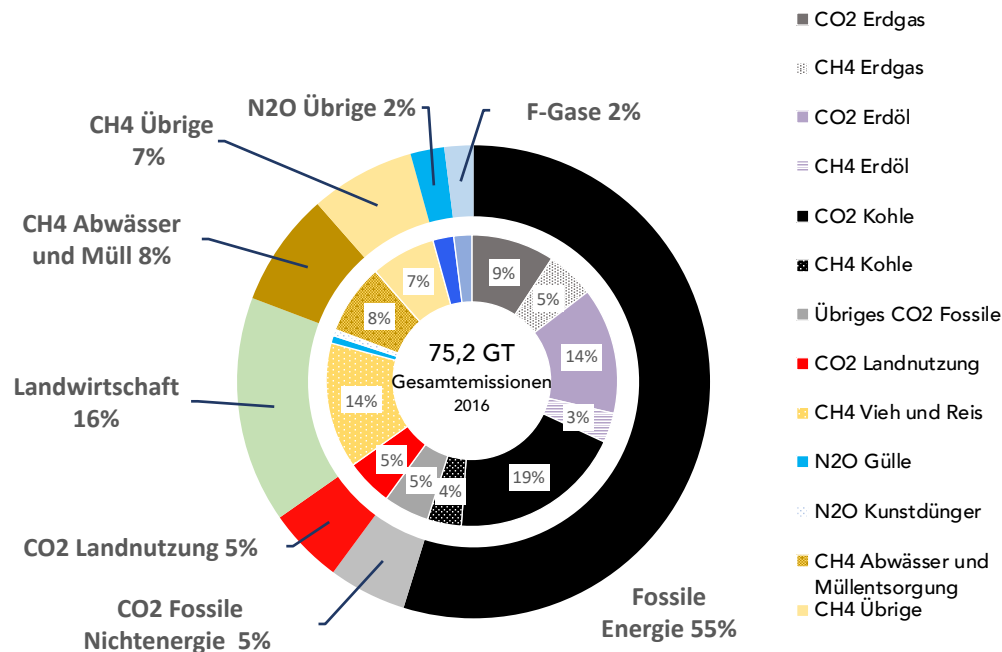
Abbildung 2: Anteil der Quellentypen an den gesamten Treibhausgasemissionen 2016: Die Emissionen fossilen Methans tragen mit einem wachsenden Anteil bei, der durch die Nutzung von Erdgas getrieben wird. EWG, 2019; eigene Berechnung auf Basis von Howarth et al. und Olivier et al. (Howarth, 2019; Olivier J.G.J. et al., 2017).
