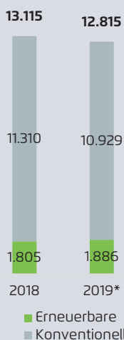
Primärenergieverbrauch (PJ)
